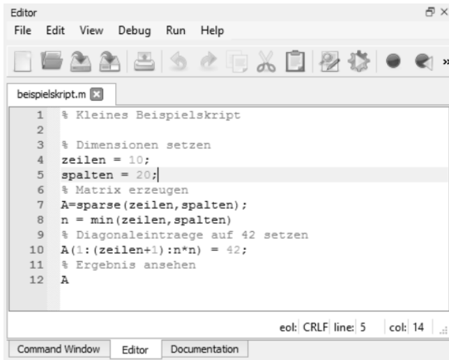
Abbildung 1.2 Screenshot Editor mit Mini-Skript (GNU Octave 4.0)
