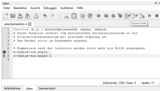
Abbildung 1.3 Screenshot: Editor im Debug-Modus (GNU Octave 4.0)
