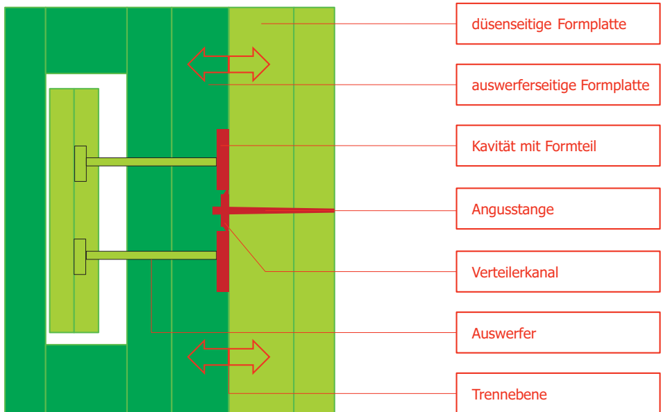
Bild 5.4 Schematische Darstellung eines einfachen Spritzgießwerkzeugs
