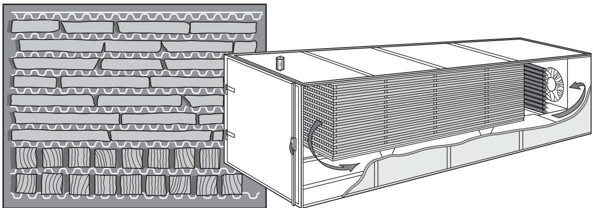
Bild 9-3 Skizze eines Kleintrockners mit Längsbelüftung. Links sind die gewellten Alu-Leisten zu sehen, die den Luftstrom längs des Stapels ermöglichen (Bild: LAUBER)
