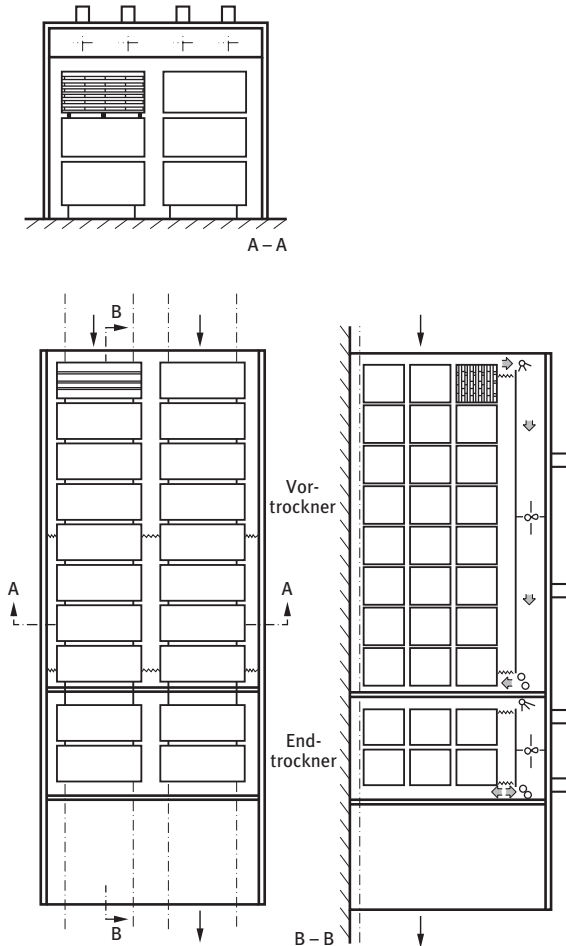
Bild 9-6 Taktdurchlauf-trockner mit Querförderung der Stapel (Prinzipdarstellung)
