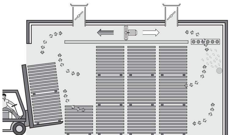
Bild 9-2 Skizze einer Großraumkammer mit Querbelüftung, beschickt mit einem Frontstapler (Bild: EISENMANN)
