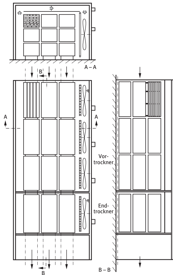
Bild 9-5 Taktdurchlauf-trockner mit Längsförderung der Stapel (Prinzipdarstellung)
