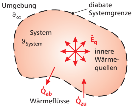
Bild 1.5: Wärmeübertragung durch Wärme-flüsse über eine diatherme Systemgrenze.
