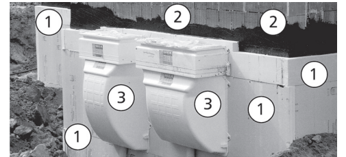
Bild 1.6: Beispiel für eine Wärmedämmung: Perimeterdämmung ① aus extrudiertem Polystyrol (XPS) an einer betonierten Kellerwand mit darüber liegender ungedämmter Ziegelwand ② sowie Aussparungen im Bereich der Lichtschächte ③. Oberhalb der Wärmedämmung ist eine Feuchtesperre in Form einer Bitumendickbeschichtung (schwarz) erkennbar, die ebenfalls keine „Isolierung“ darstellt.
