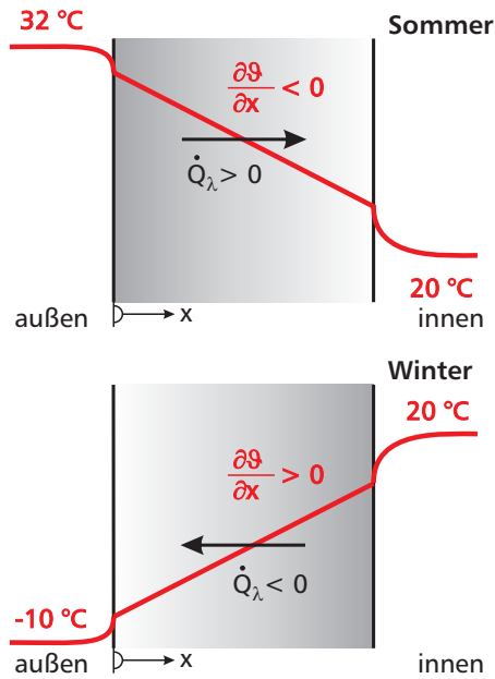
Bild 1.11: Stationäre Wärmeleitung in einer Außenwand mit beidseitigem Wärmeübergang (oben: im Sommer; unten: im Winter).
