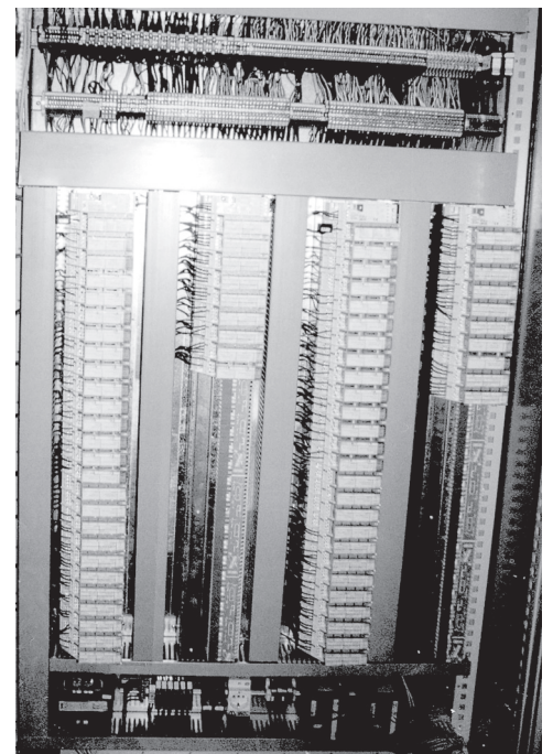
Bild 1.4: Elektrischer Schaltschrank.
