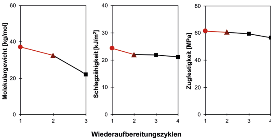
Bild 3.3 Gewichtsgemitteltetes Molekulargewicht und mechanische Eigenschaften von Roh-Polyethylenterephthalat (PET) und wiederaufbereitetem PET, in Abhängigkeit der Anzahl der Wiederaufbereitungsschritte (Extrusion) [34]
