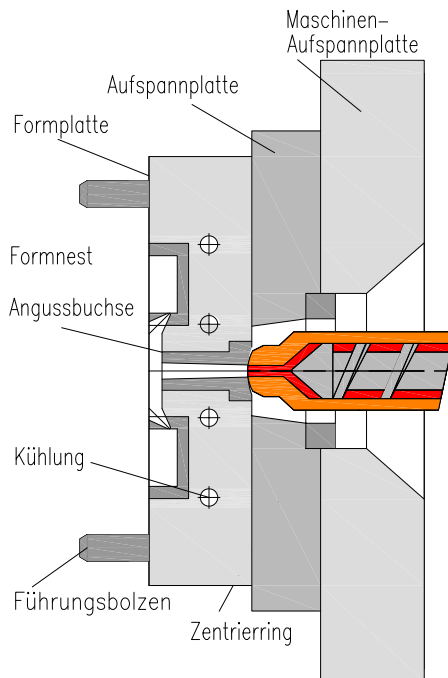
Bild 1.2 Düsenseitige Werkzeughälfte
