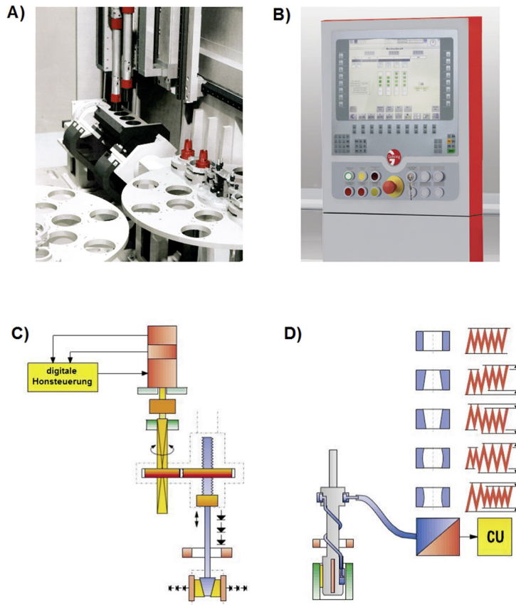
Bild 1.4 Hontechnik um 2019 (nach Gehring) Endbearbeitung von Bohrungen durch Honen A) Modulares Honzentrum mit automatischem Werkzeugwechsel-System B) Digitale Honsteuerung mit bedienerfreundlichen dezentralen Stationspulten C) Elektromechanische Schrittzustellung mit Kraftsensorik D) Pneumatische In-Prozess-Messung mit Maß- und Formregelung
