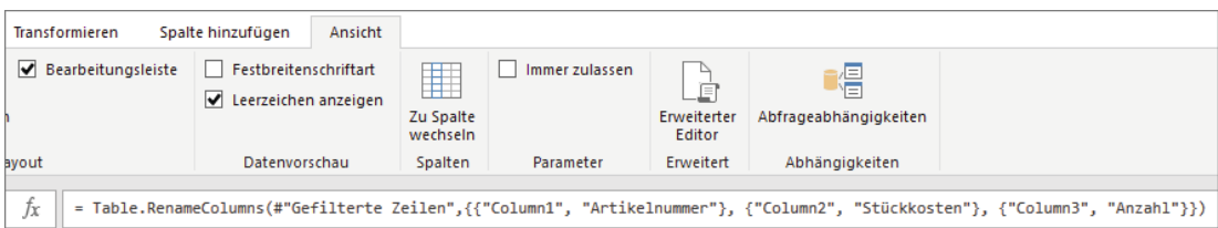
Bild 10.1 Die Bearbeitungsleiste zeigt den M-Code des aktiven Schritts an.
