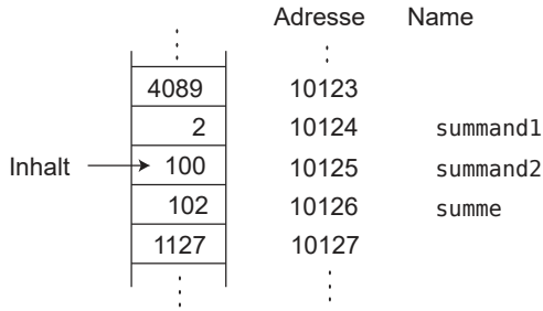
Abbildung 1.1: Speicherbereiche mit Adressen
